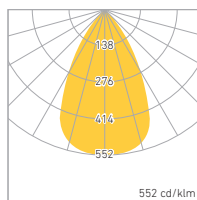
REFLECTOR 50°
