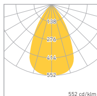
REFLECTOR 50°
