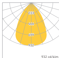
REFLECTOR 90°
