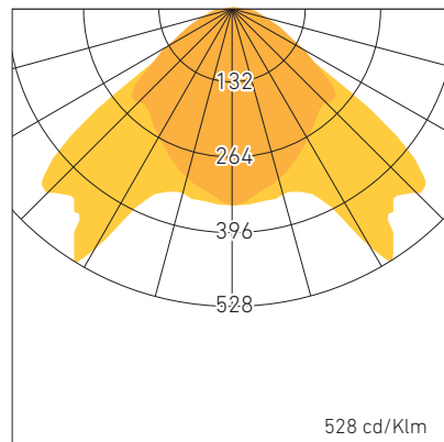
5.1 EFICIENCIA DEL SISTEMA 90 lm/W
